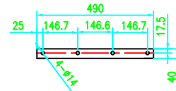
件9 短法兰6厚, 2件
